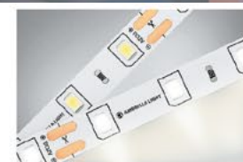
GS1002 белый 5000*8*1.2 LED 4,8 Вт/мW IP20 4500K дневной белый свет 663 p.
