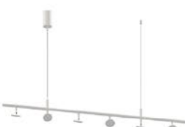
C9005 белый песок 1200*60*H1200 GU5.3*6 max 12W IP20
