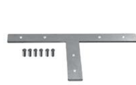
GP8055 серебро 100*55*1,55 Соединитель угловой Т для профиля Profile System 459 р.
