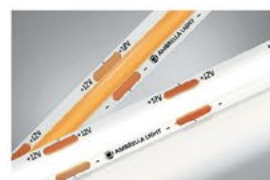
GS2602 белый 5000*8*1.54 LED 10 Вт/мW IP20 4500K дневной белый свет 1 683 р.
